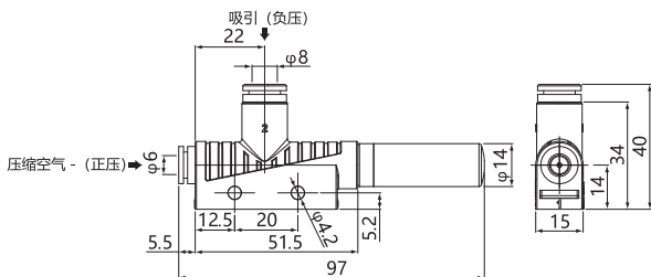
塑料真空发生器 喷嘴2.0mm
