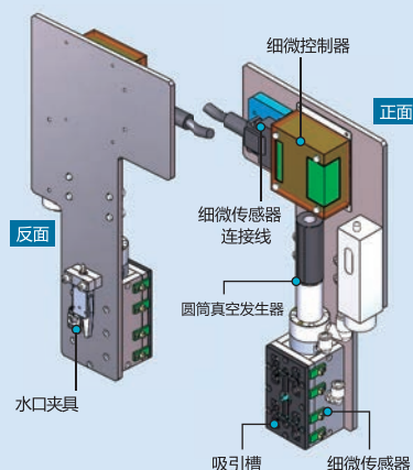
细微型夹具案例 ※总重量：900g
