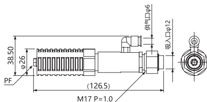
消声器
